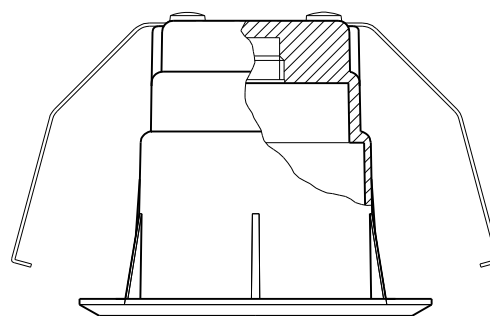
埋込カバー
