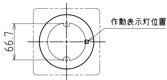
取付寸法図
