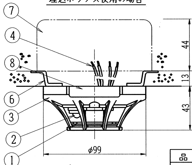
埋込ボックス使用の場合
