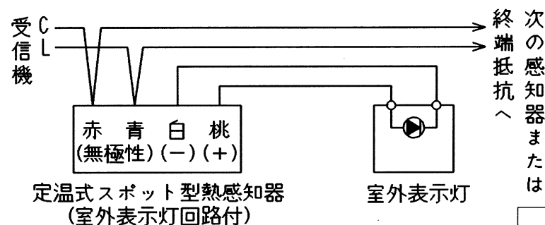
接 続 図
