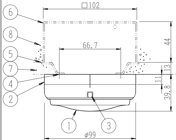
埋込ボックス使用の場合
