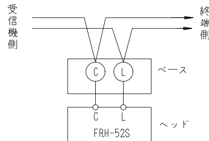
FRH-52S接続回路図
