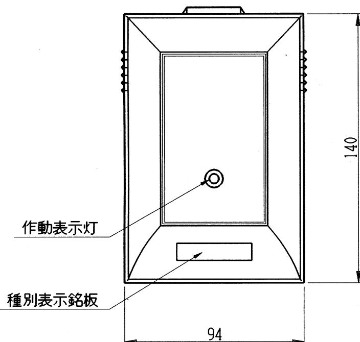
通線孔及び取付孔位置 (正面図)
