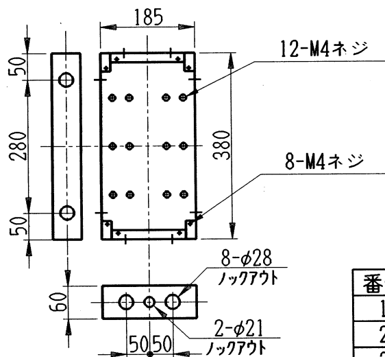
取付寸法図
