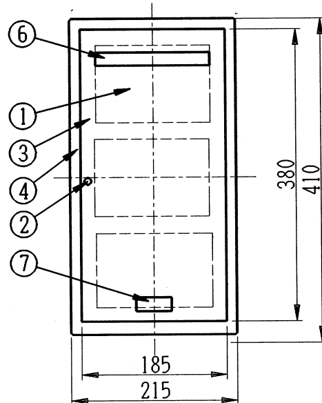
取付寸法図
