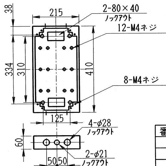
取付寸法図
