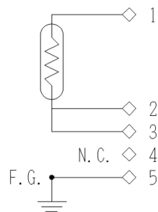
内部結線図
